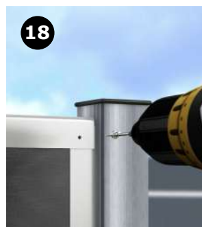
18 Skru skruer i hvor hullerne tidligere blev lavet, her skrues også igennem hegnsp profileren
